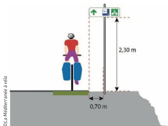
Implantation en hauteur
